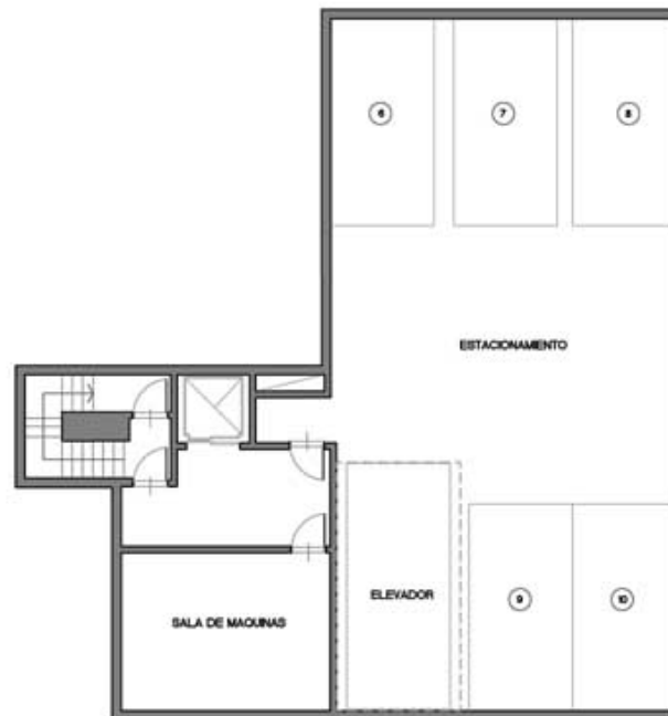
2do. SUBSUELO
